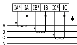
交流电流(>10A时)互感器接入
