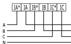
交流电流(≤10A时)直接接入
