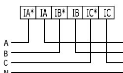
交流电流(≤10A时)直接接入
