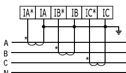
交流电流(>10A时)互感器接入
